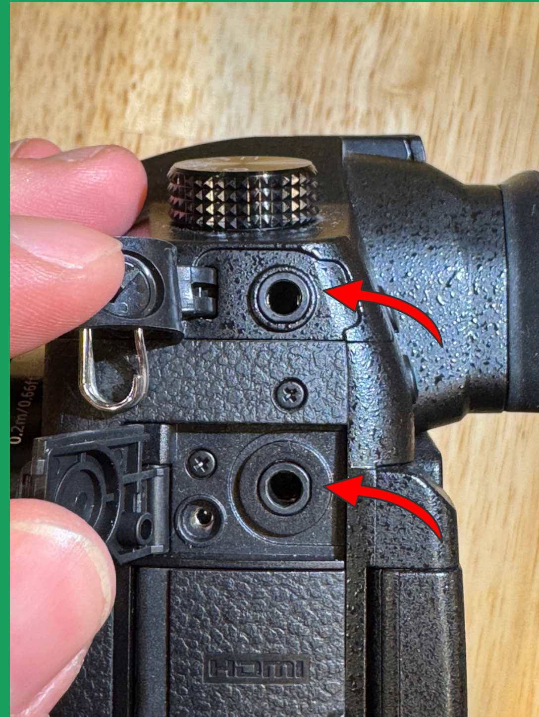
(上) 送信機のラインを差し込む
